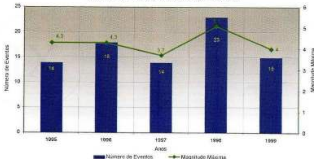
Gráfico 8.20 - EVOLUÇÃO DO NÚMERO ANUAL DE SISMOS BRASILEIROS COM MAGNITUDE MAIOR OU IGUAL A 3,0 - 1995-1999
