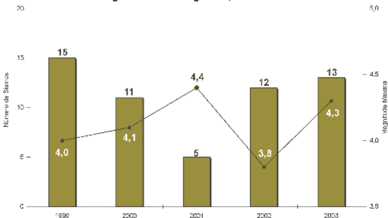
Gráfico 8.18 – Evolução do Número Anual de Sismos Brasileiros com Magnitude Maior ou Igual a 3,0 – 1999–2003
